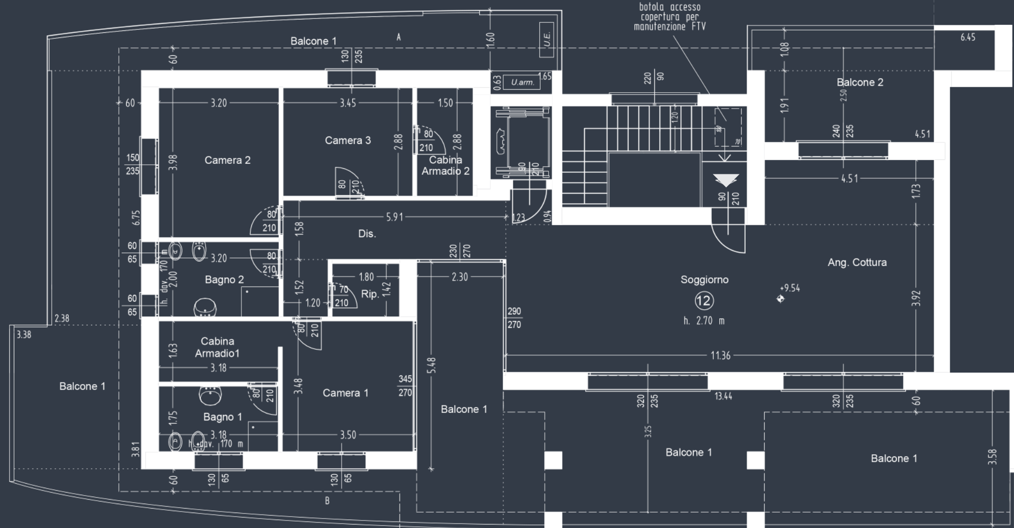
PIANO TERZO
